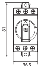
Рисунок 2. Габаритные размеры РМ (мм)
