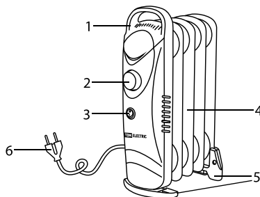
Рисунок 1. Устройство масляного обогревателя
