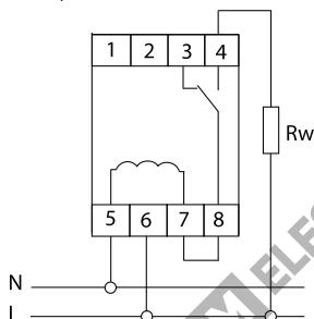
Рисунок 3. Схема подключения ограничителя мощности OM-3 к сети (при нагрузке менее 2 кВА)
