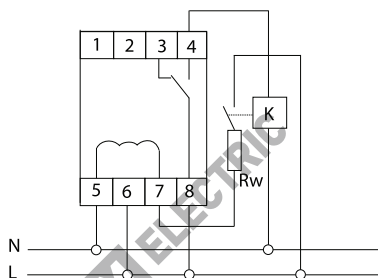
Рисунок 4. Схема подключения ограничителя мощности OM-3 к сети (при нагрузке более 2 кВА с использованием контактора)
