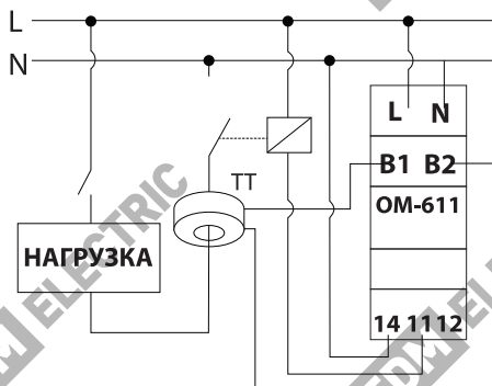
Рисунок 5. Схема подключения OM-611 к сети
