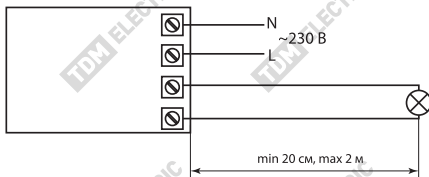
Рисунок 1. Схема подключения.
