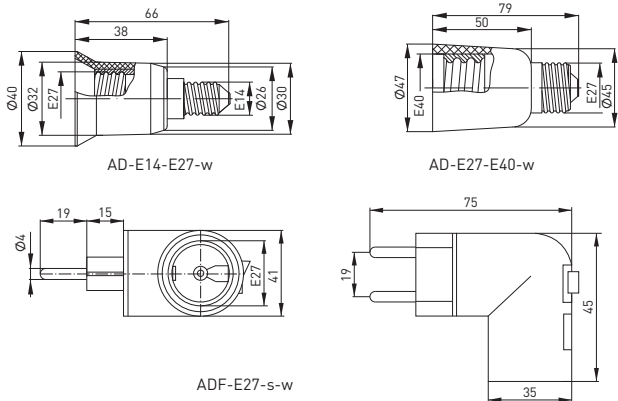
Рис. 5 – Адаптеры-переходники
