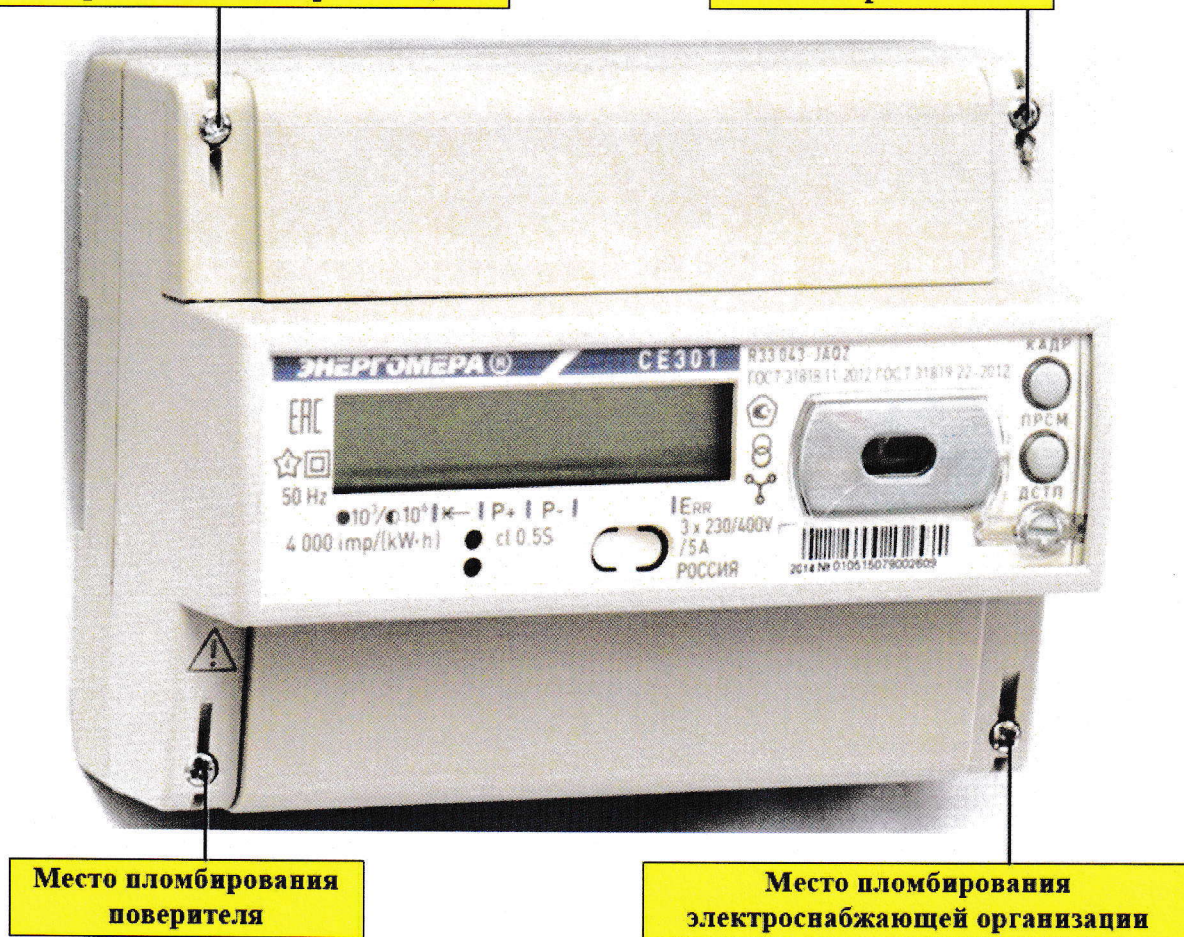
Рисунок 2 – Общий вид счетчика CE301 R33
