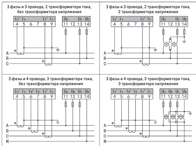
Рис. 5 Схема подключения
