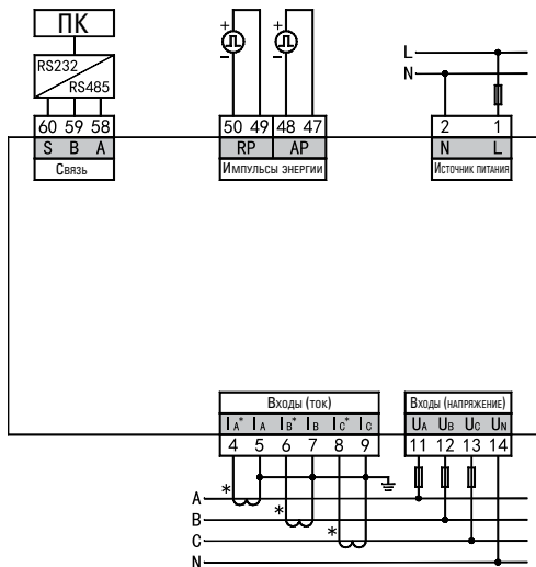
Рис. 4 Расположение клемм
