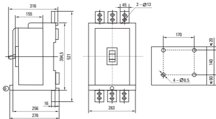
Габаритные и установочные размеры ВА-99М 1250А
