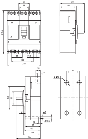
Габаритные и установочные размеры BA-99M 800-1000A*
