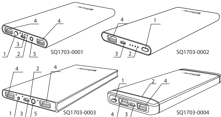
Рисунок 1. Конструкция аккумуляторов
