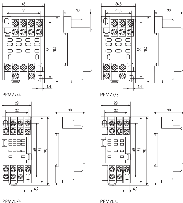
Рисунок 1. Габаритные размеры, мм
