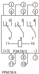
Рисунок 2. Схемы подключения
