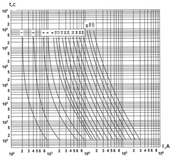
Рис. 2 Времятоковые характеристики ПВЦ
