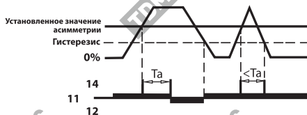
Рисунок 7. Схема работы реле РН (кроме моделей РН-04, РН-05) при асимметрии фаз
