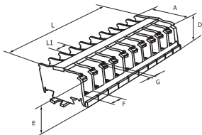
Клеммный терминал серии ТК
