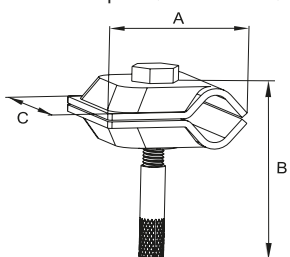
Зажим прута универсальный с анкером (M8 x 30 мм)
