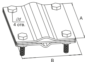
Зажим прута универсальный с анкером (M8 x 30 мм)
