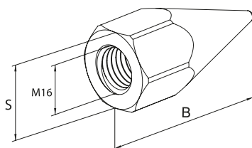
Наконечник заземлителя
