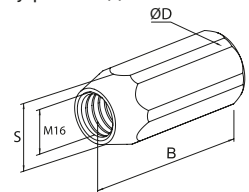
Гайка переходная
