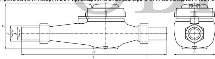
Приложение А. Габаритные и присоединительные размеры счетчиков холодной и горячей воды СВМ
