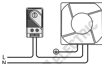
Рисунок 1. Наглядная схема подключения термостата с вентилятором
